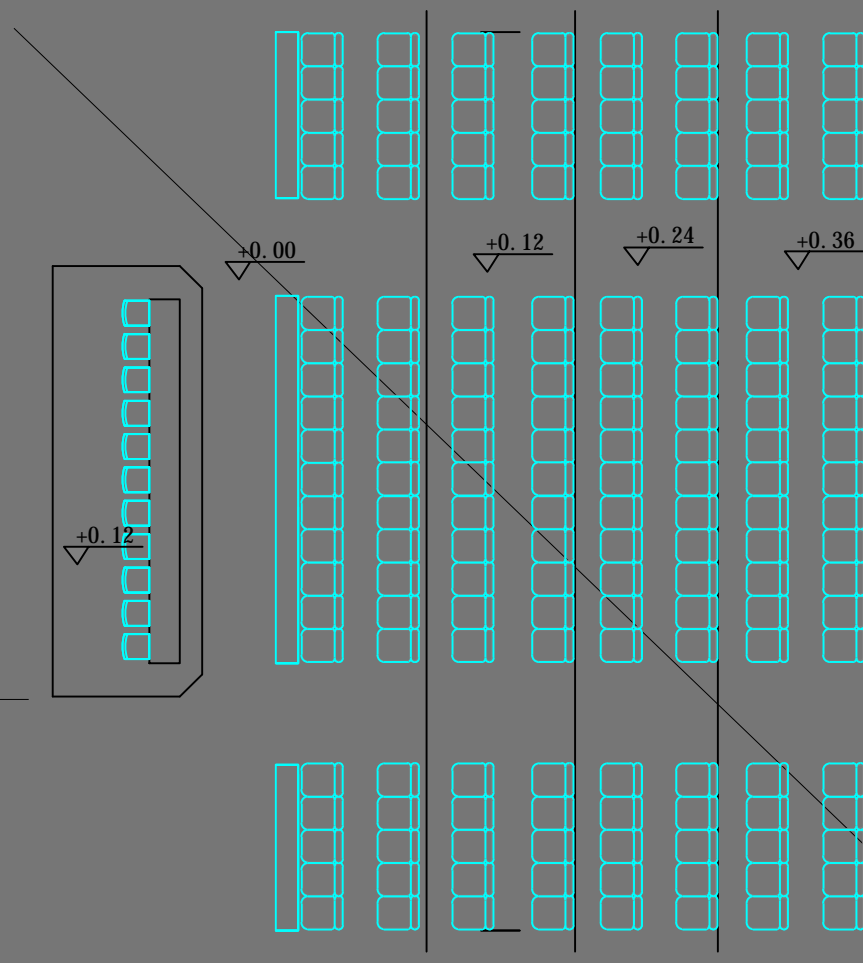
桐城师范高等专科学校教学楼东阶梯教室会议室顶面图
