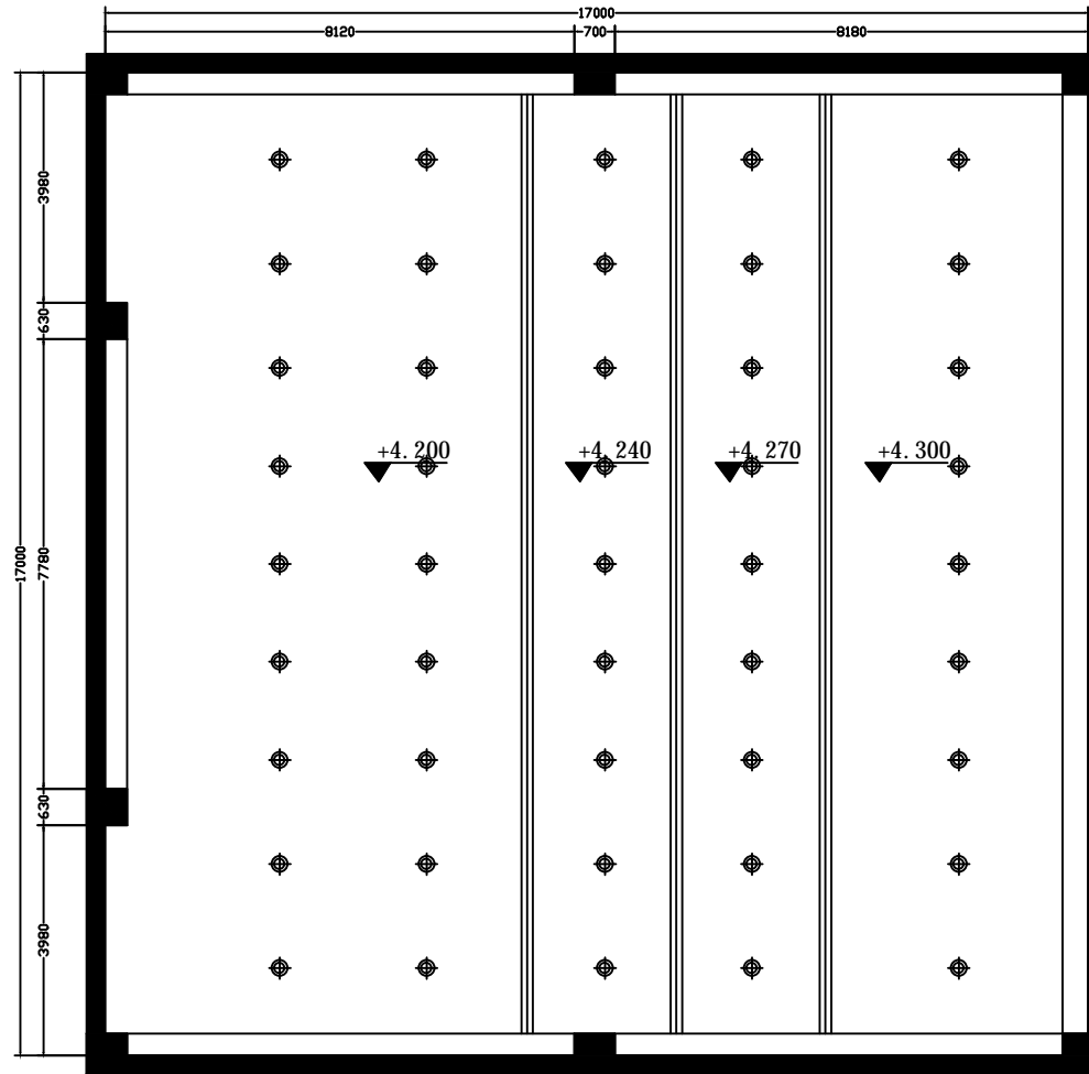
桐城师范高等专科学校教学楼东阶梯教室会议室顶面图
